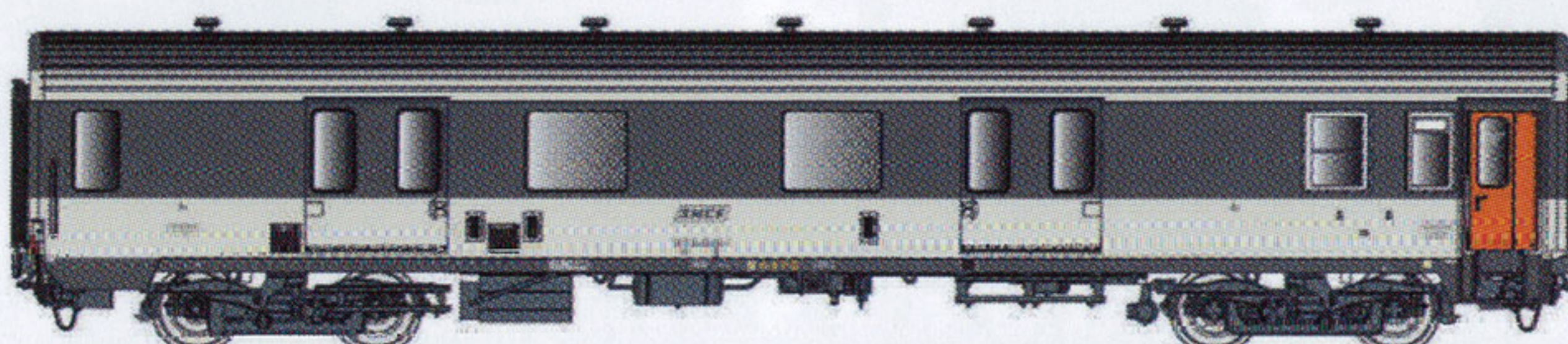
31 231 Fourgon MC 76 Dd2 Livrée Corail, Logo Encadré Ep IV.
